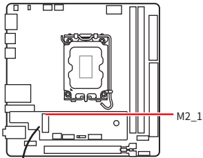
マザーボードの上面図
