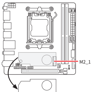
マザーボードの上面図
